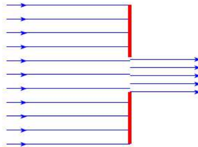
Grande ouverture = pas de diffraction
